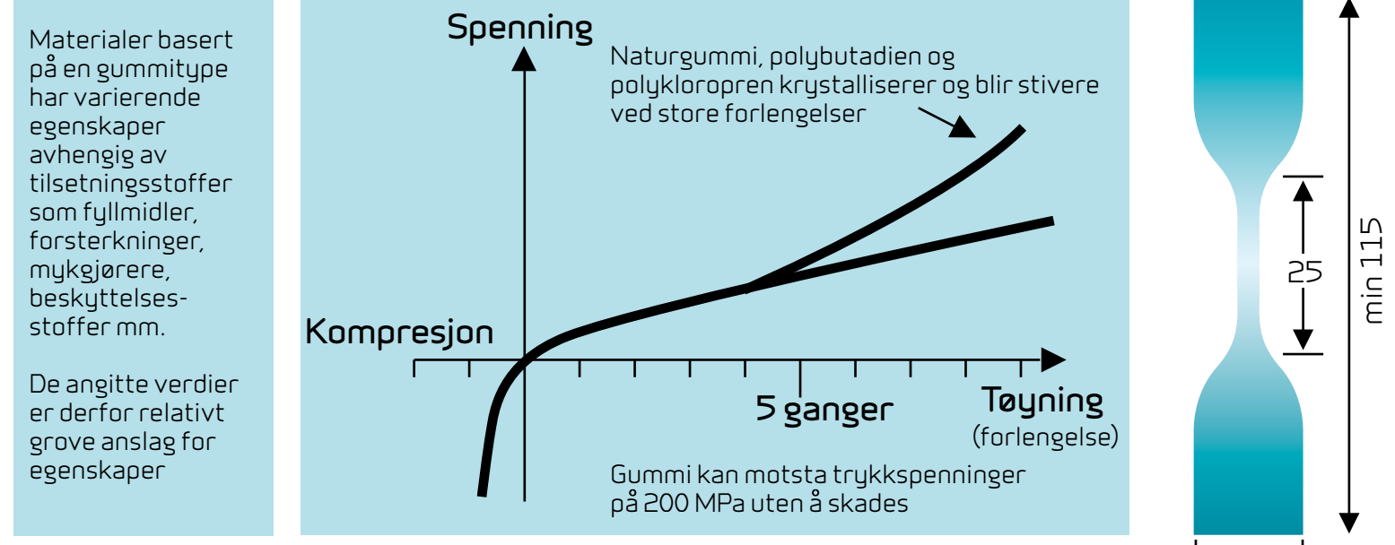
PRØVESTYKKE FOR GUMMI Tykkelse 2mm. Stivhet er vanligvis gjengitt med strekkstyrke i tøyning på 100%, 200%, 300% osv
